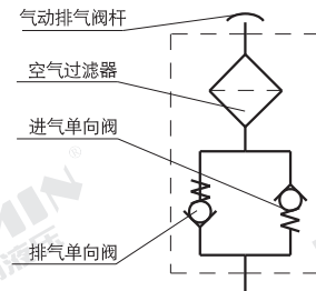
符号及工作原理图 Circuit symbol
